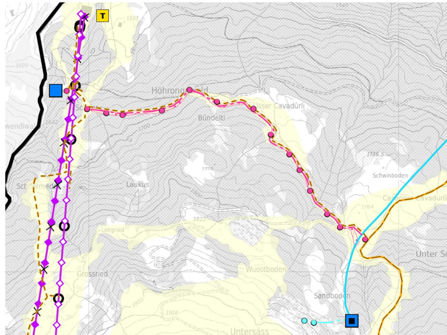
Abbildung 10: Übersicht geplante technische Beschneuerung zwischen Casanner Cavadürli und Schifer (Quelle: GeoGR, massstabslos)
