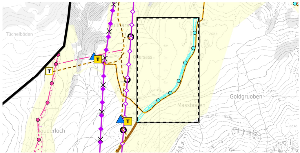
Abbildung 12: Anpassung technische Beschneidung im Bereich «Mässboden» und Fenster mit aufhebender Wirkung (massstabslos)
