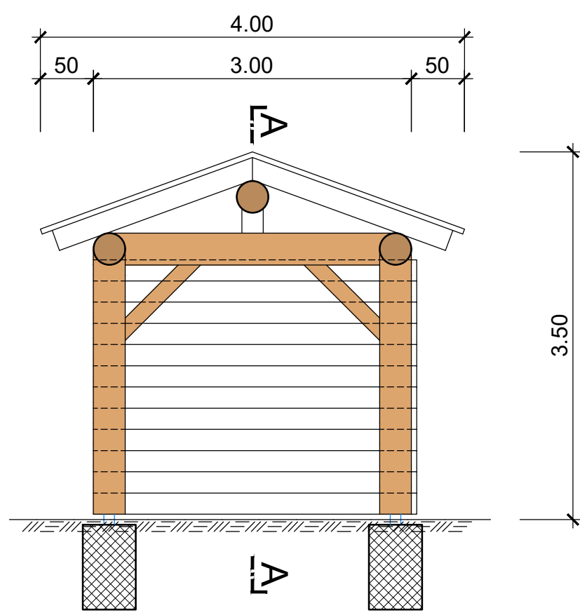
Schnitt B-B 1:50
