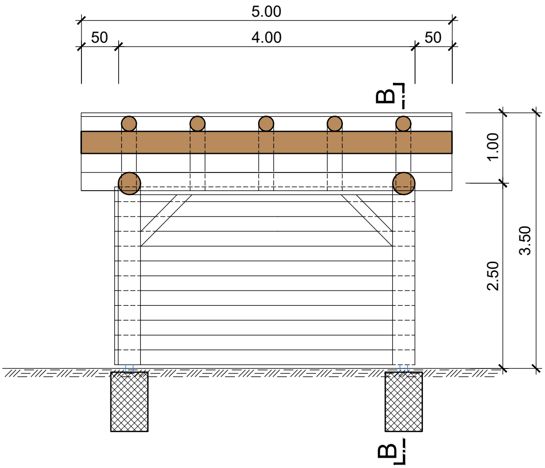
Schintt A-A 1:50
